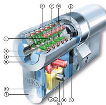
Veiligheidscilinder met boorbeveiliging (foto BKS)
